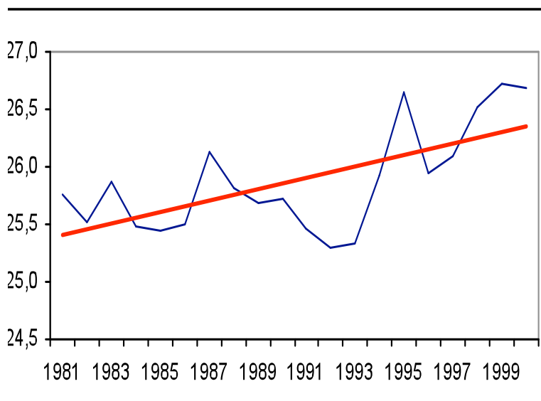
Figura 6. Tendencia temperatura promedio anual en la Cuenca del Haina. Serie 1981 -
